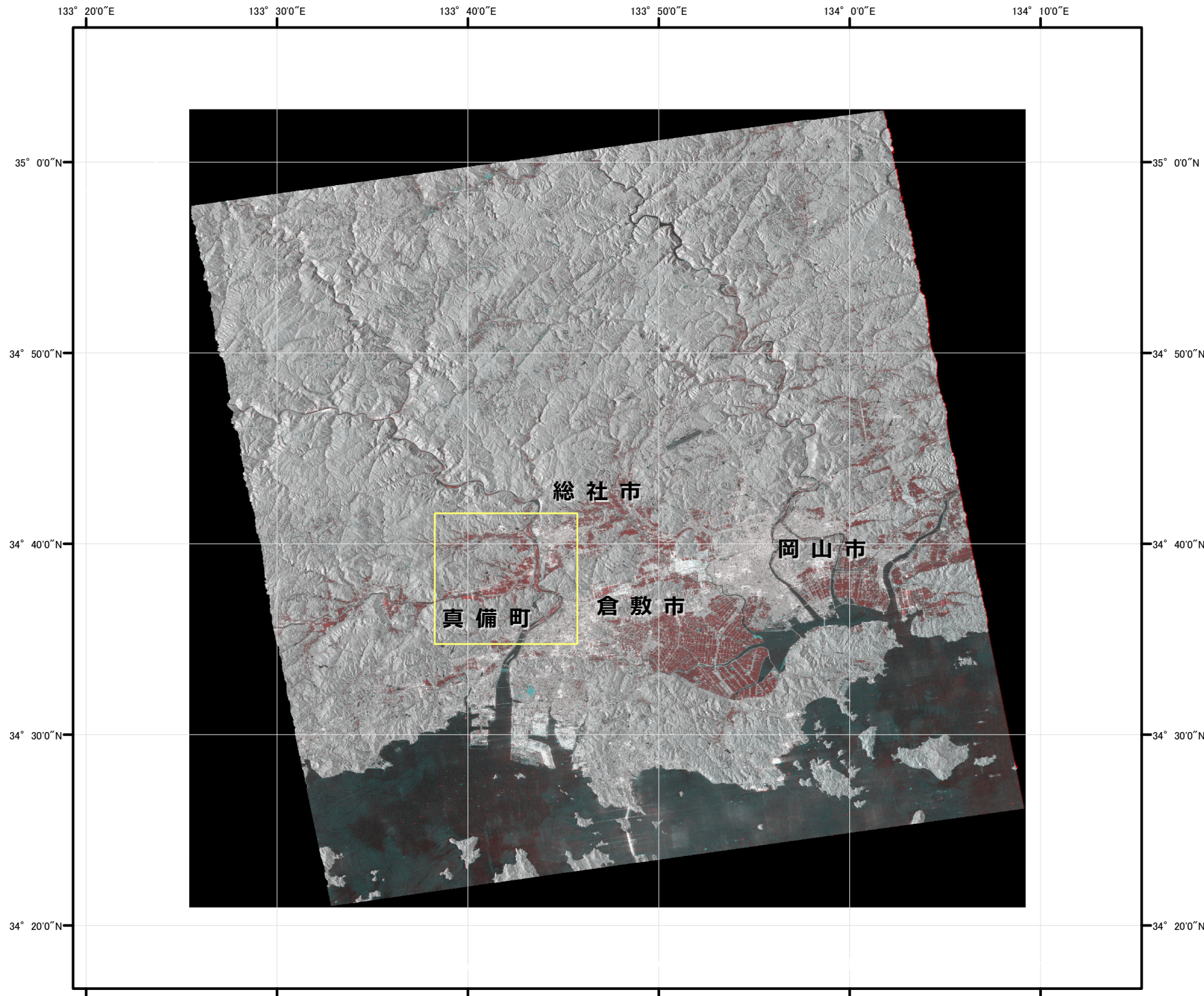
ALOS-2/PALSAR-2 image (R: 2018-04-14, G & B: 2018-07-07)
